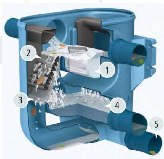
Coupe du VF1 Twin
