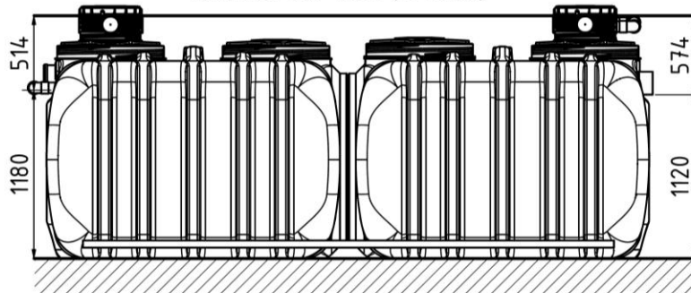
Actibloc 185 18EH (bi-cuve)
