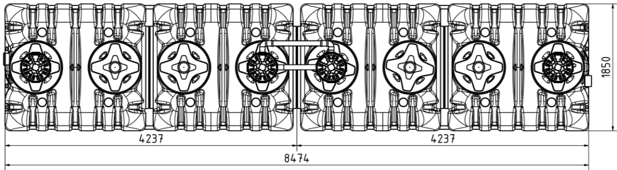
Actibloc 185 18EH (bi-cuve)
