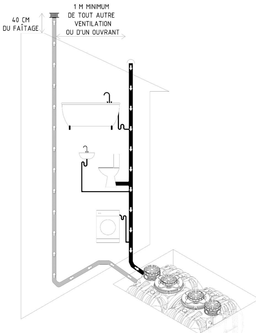
Figure 5 – Vue schématique de la ventilation ACTIBLOC 185 4 EH
