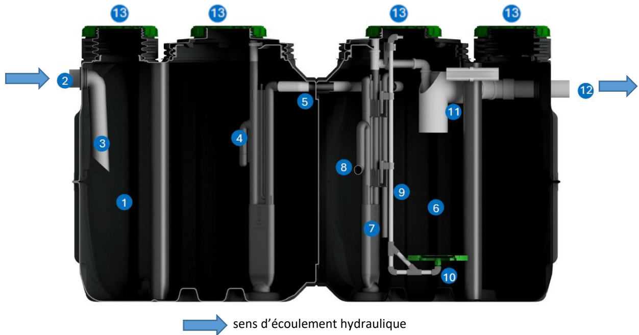
Figure 1 - Schéma de principe de la filière ACTIBLOC® 185 4 EH
