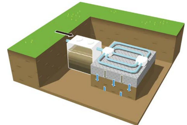
Lit d'épandage
