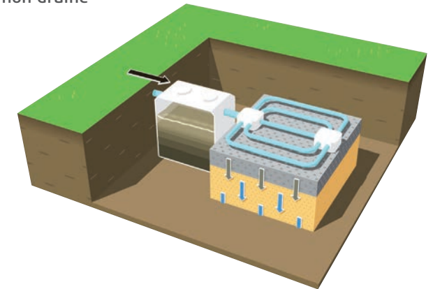
Filtre à sable vertical non drainé
