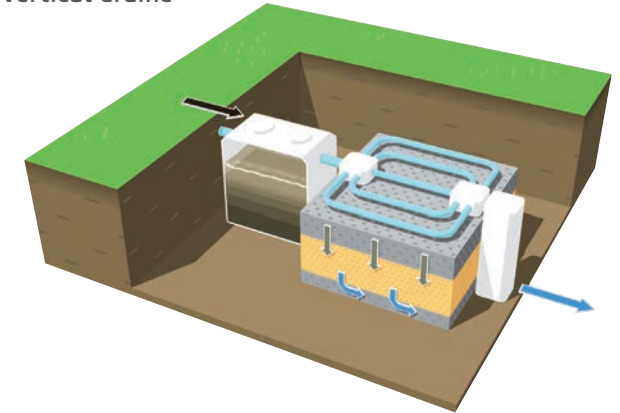
Filtre à sable vertical drainé
